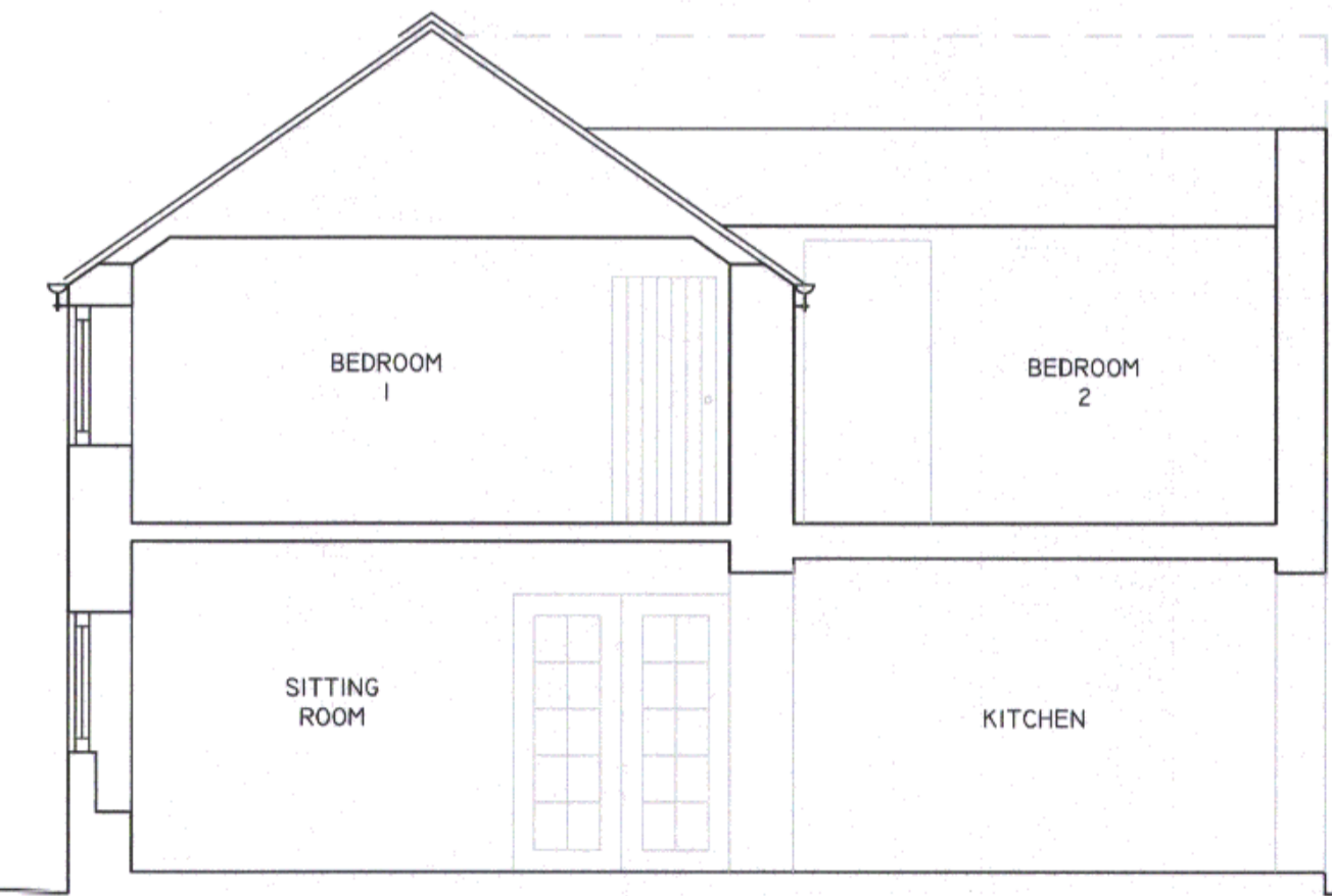
AA SECTION LATITUDINAL 1:50
