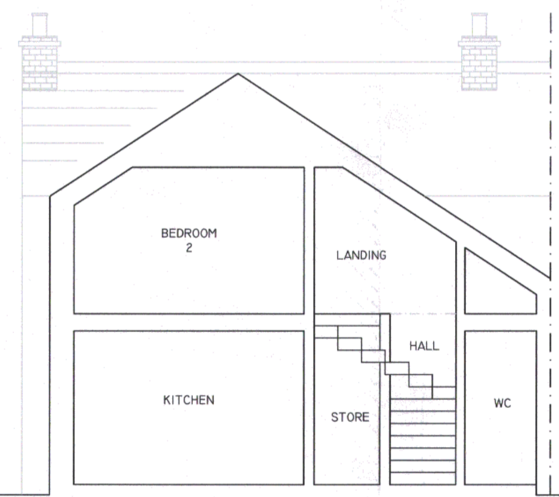
BB SECTION LONGITUDINAL 1:50
